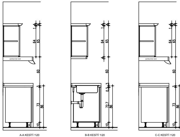
MUTFAK DOLABI KESİTLERİ ÖLÇEK 1:20
