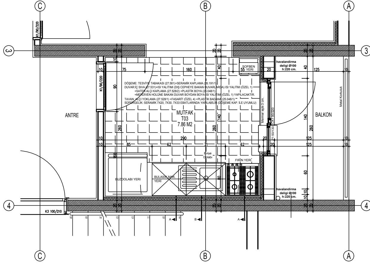
MUTFAK PLANI ÖLÇEK 1:20
